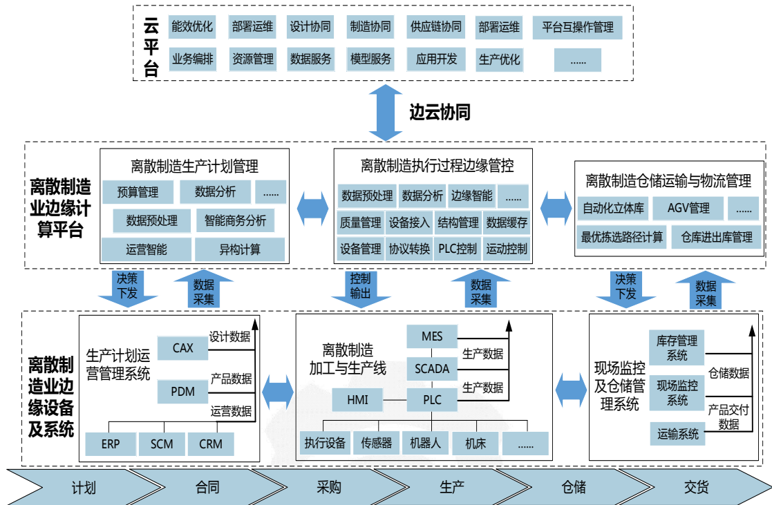
图 2 离散制造业边缘计算实施参考架构
