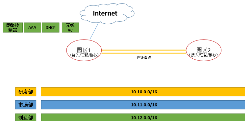
图 2 本地多园区虚拟化网络组网拓扑
