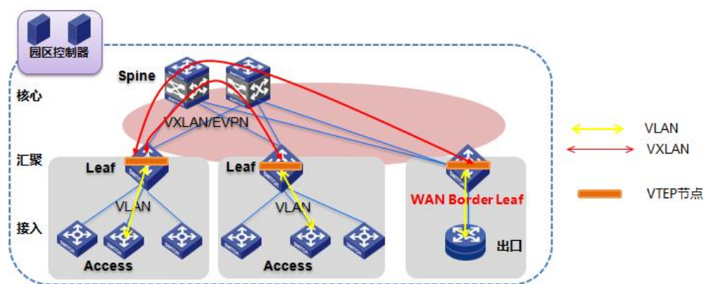
图 8 大二层网络架构
