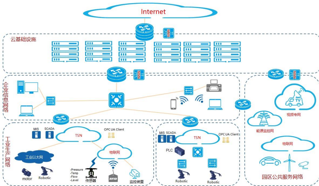
图 5 工业互联网园区网络总体架构
