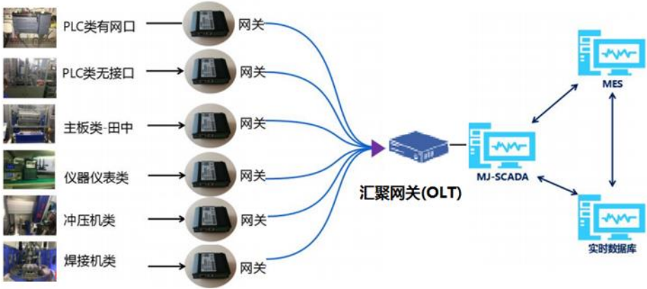
图 25 工业 PON 组网架构
