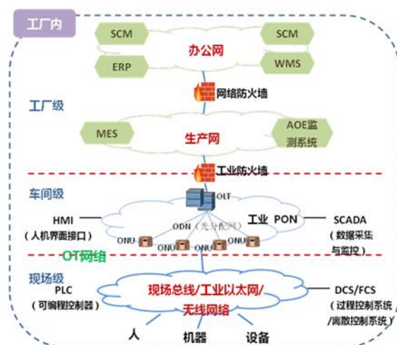
图 24 工业 PON 在工业互联网架构中位置
