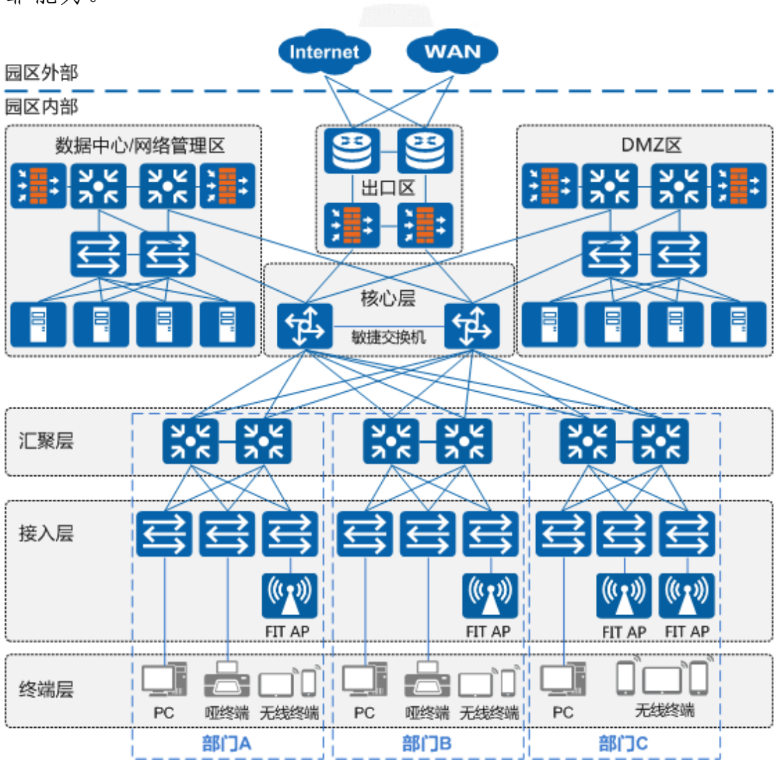
图 13 基于融合交换机的有线无线融合解决方案
