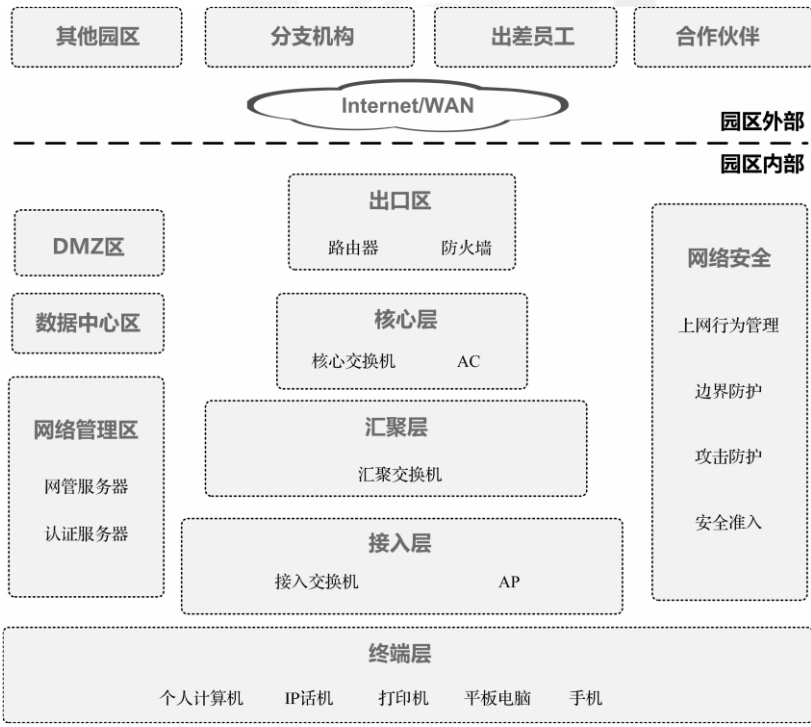
图 7 三层（核心、汇聚、接入）架构 + 传统 VPN
