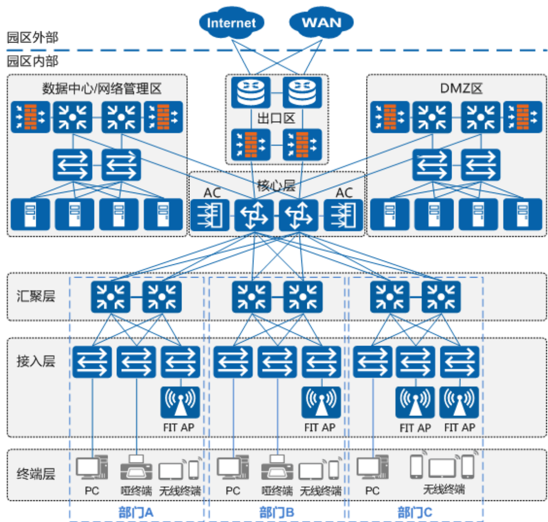
图 11 大型网络的 Wi-Fi 组网架构
