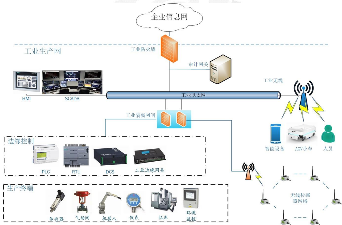
图 4 工业生产网络架构
