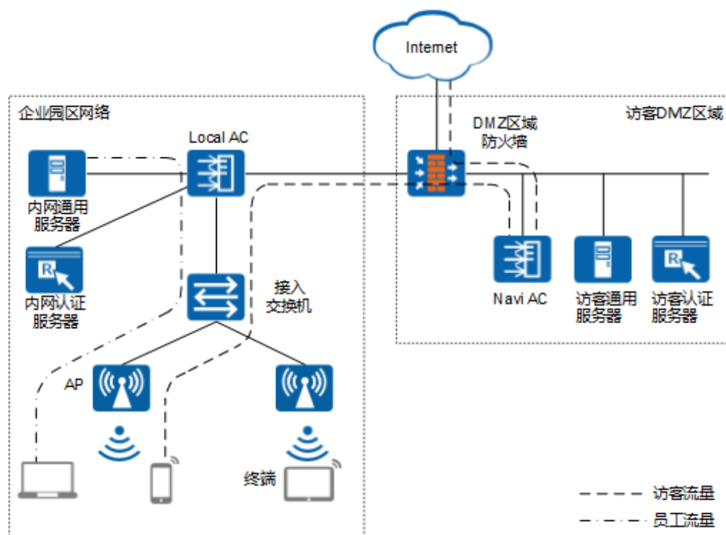
图 12 NaviAC 典型组网
