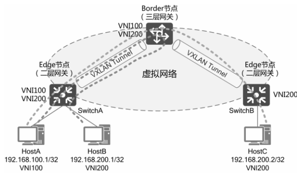
图 19 集中式网关示意图
