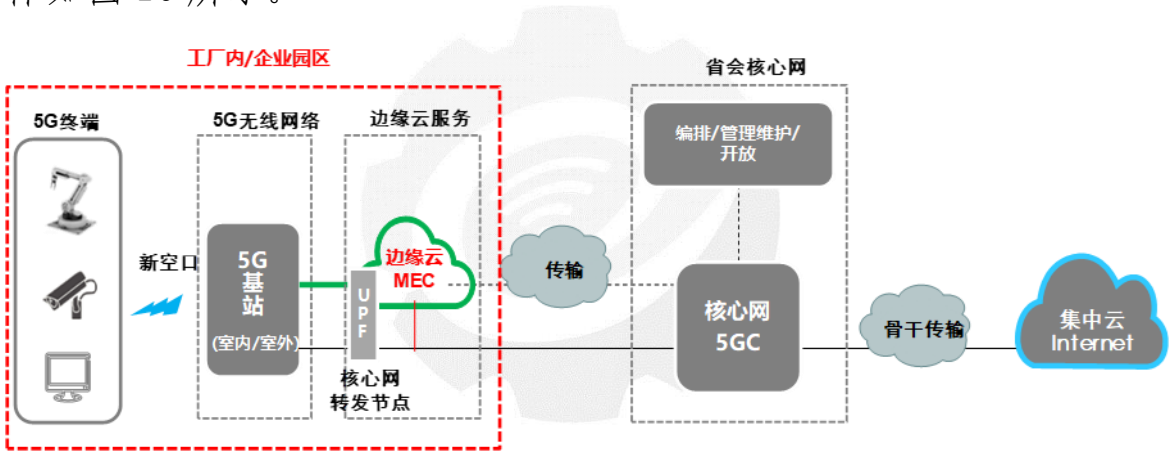
图 26 5G 园区网络部署
