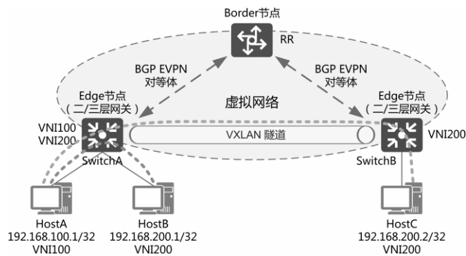
图 20 分布式网关示意图
