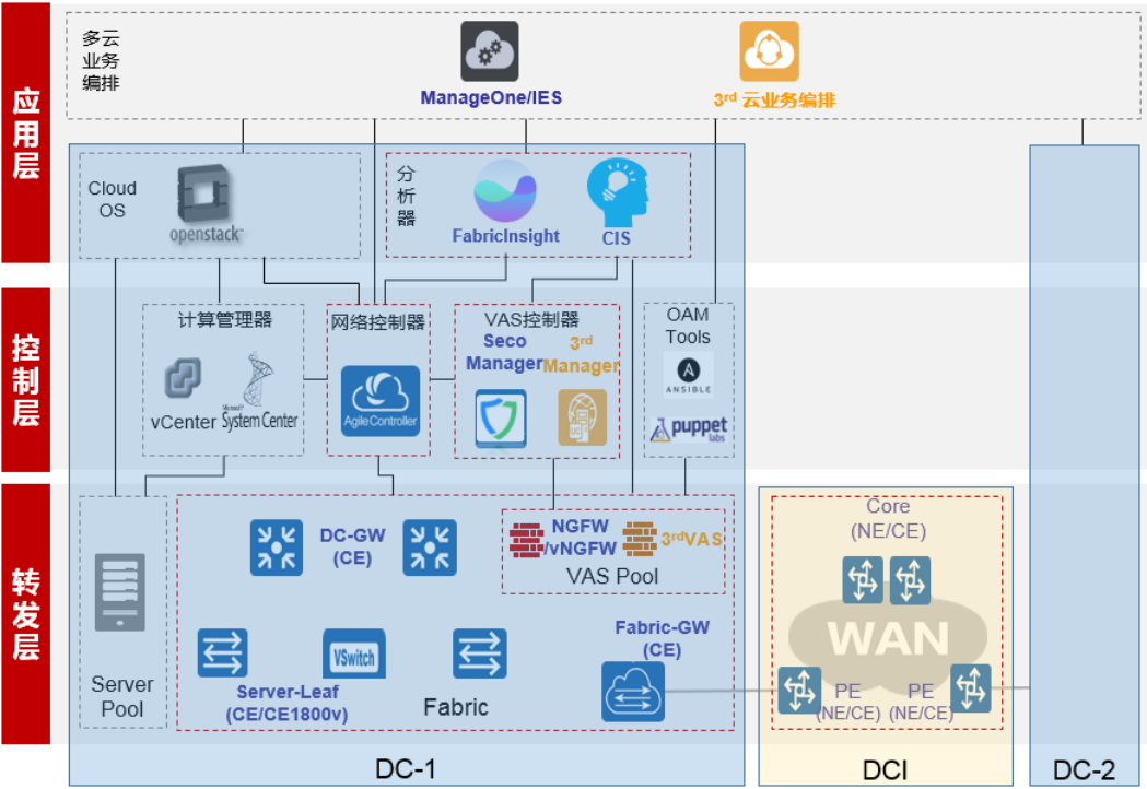
图 6 数据中心架构
