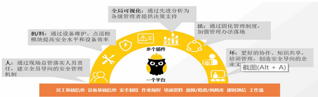
图 22 移动 HSE
