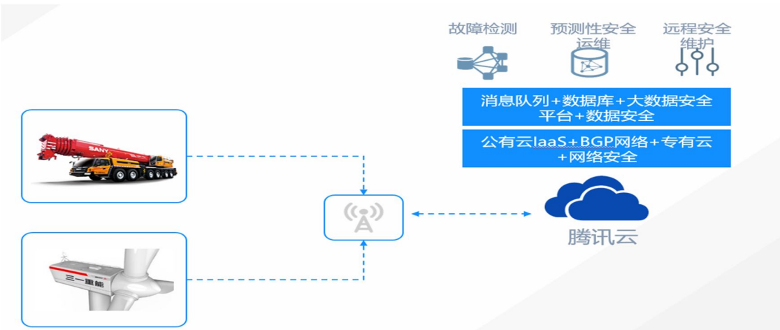
图 17 安全能力
